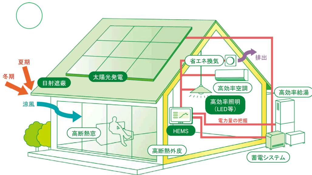
図 24 ZEHの概念図 (イメージ) 出典：資源エネルギー庁ホームページ
