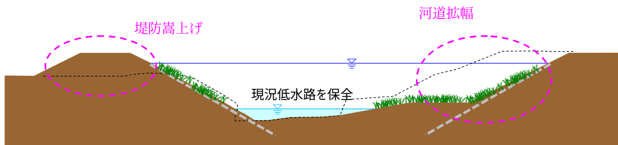
図－4.2 赤川河川整備計画 (横断概要図)
