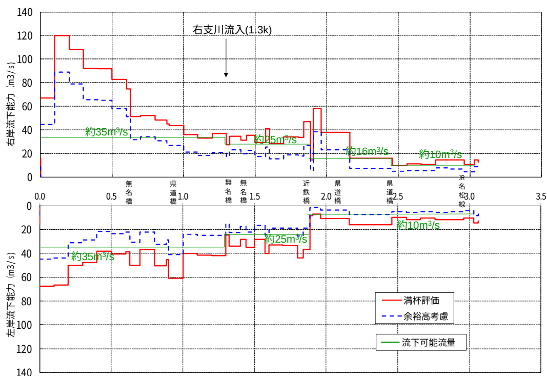
図－2.4 赤川現況流下能力図
