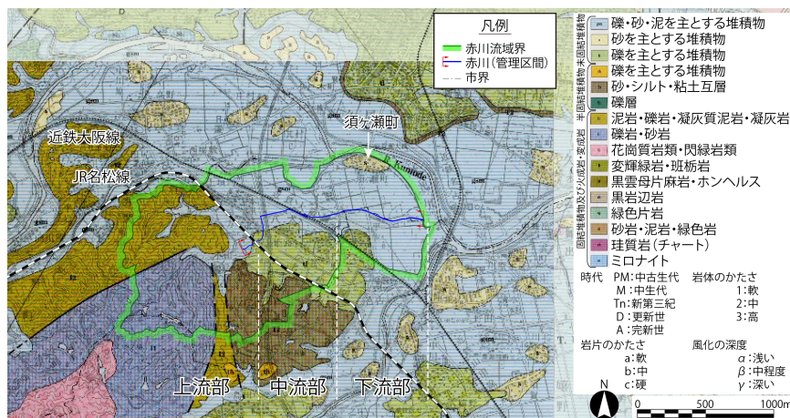
図-1.4 地質図
