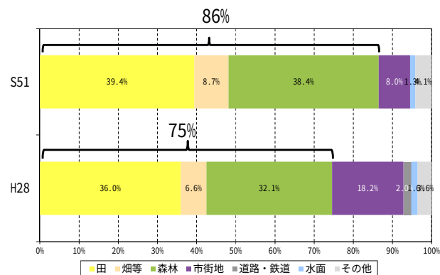
図- 1.10 赤川の土地利用図と土地利用別の面積割合の変化
