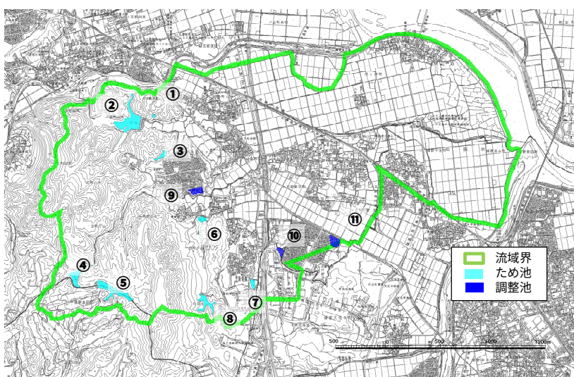
図-4.3 赤川流域のため池等
