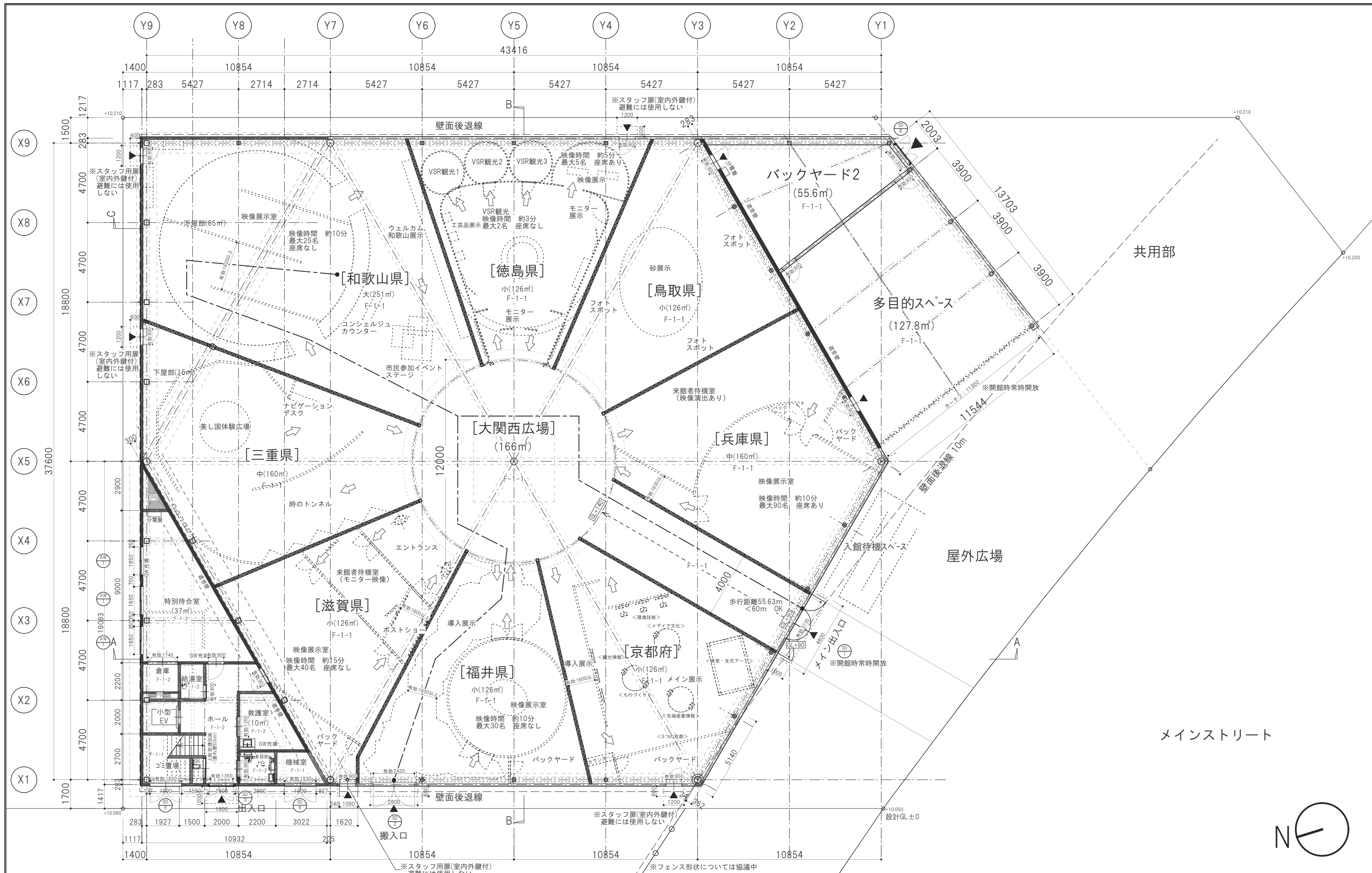
一級建築士 大臣登録第242899号 野口 明裕 配置図兼 1階平面図
