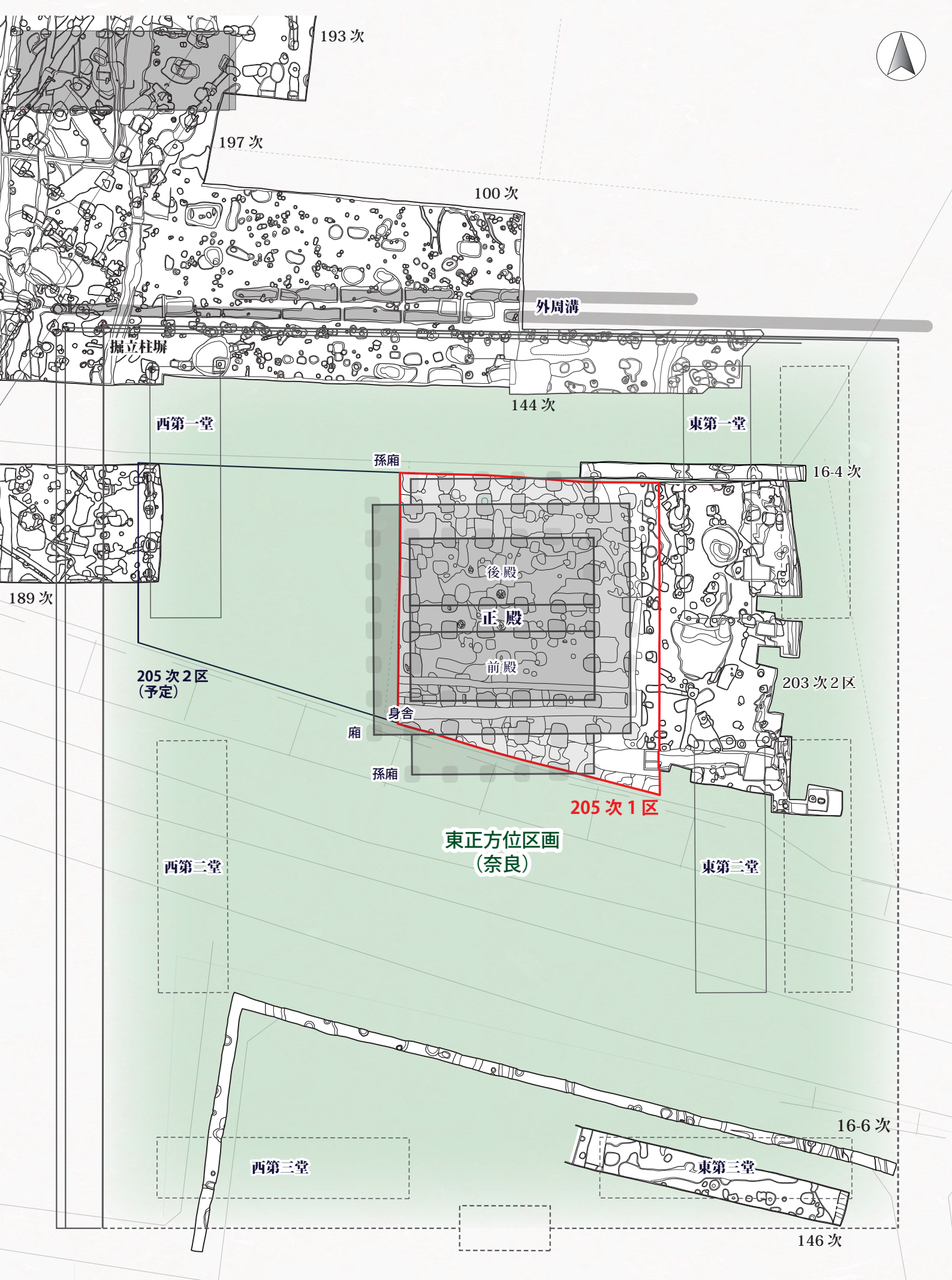
東正方位区画の遺構配置図 (推定復元)
