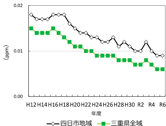
図 2-4-2 二酸化窒素の経年変化（一般局の年平均値）
