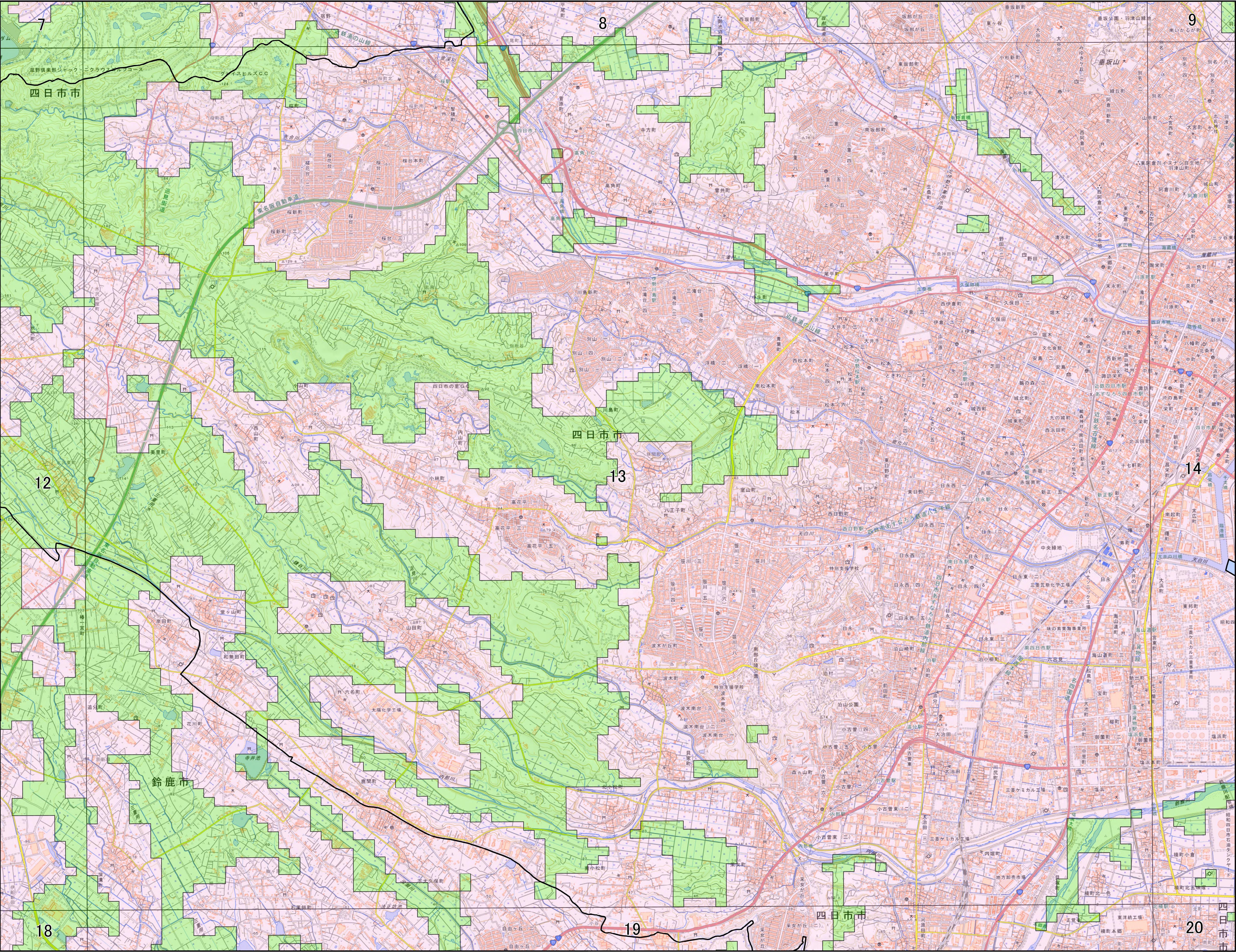
宅地造成及び特定盛土等規制法に基づく規制区域 詳細図 13
