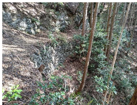
図 117 三浦峠道 野面乱積みの石垣
