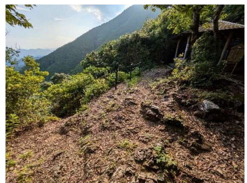
図 37 ツヅラト峠に露出した岩盤
