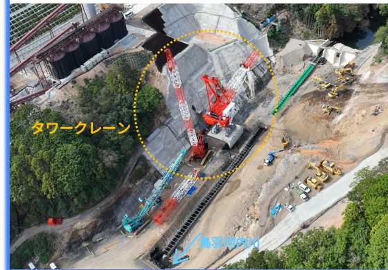
①ダム本体工事 タワークレーン
