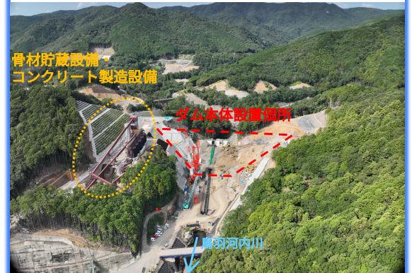
①ダム本体工事 施工状況（全景下流側より）
