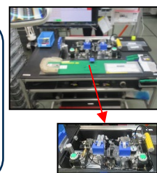
収納式リブカット機を内蔵
