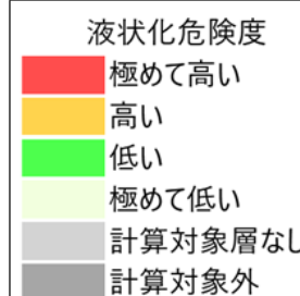
<液状化危険度別面積割合>
