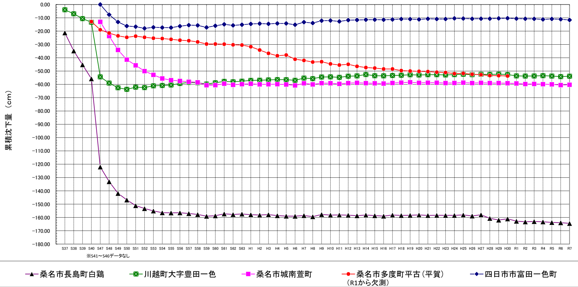
図-1 主な水準点の経年変化
