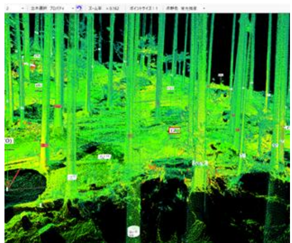
3次元点群測量による流木発生状況の調査
